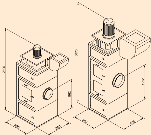
FILTERCUBE 4N (izquierda) y FILTERCUBE 4H (derecha)
