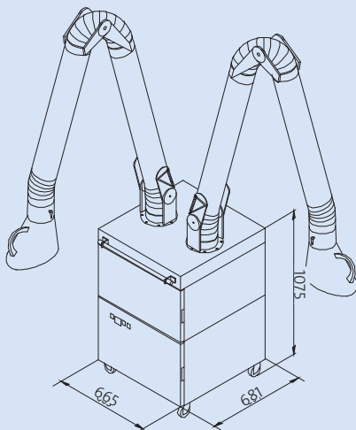
CAREMASTER-IFA (Número de art. 97 320 111)
