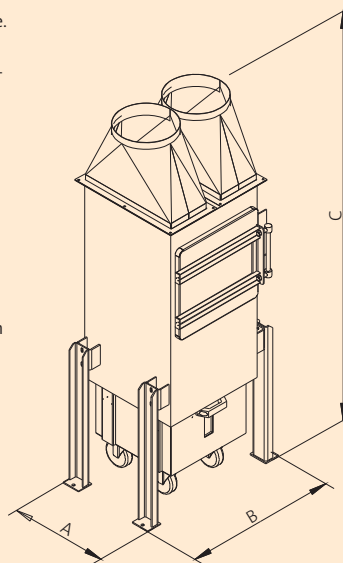
Pre-separador de chispas
