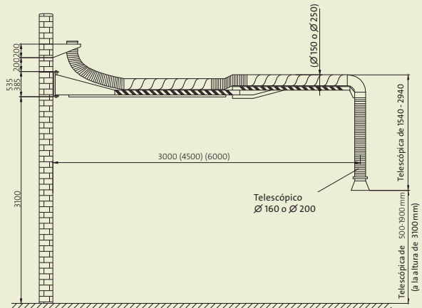
Grúa de Aspiración (Número de art. 97 641)
