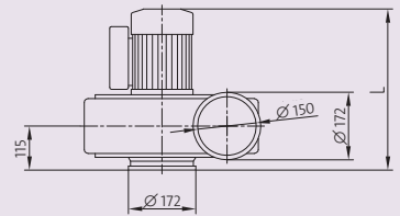
Aspirador de siluminio fundido
