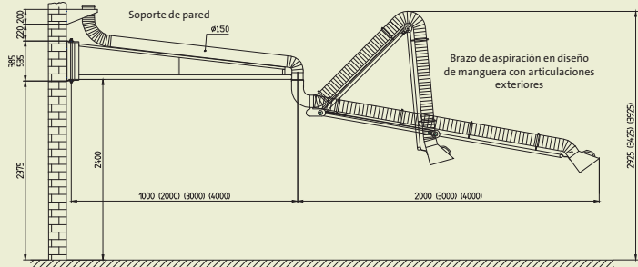
Brazo de aspiración (Número de art. 97 631)
