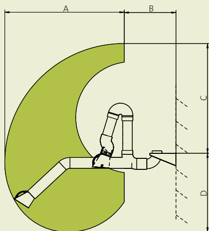
Brazo de aspiración (Número de art. 97 621)
