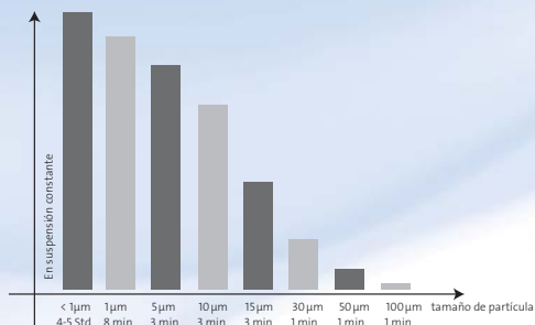
Gráfico de barras: Tiempo de sedimentación de las partículas
