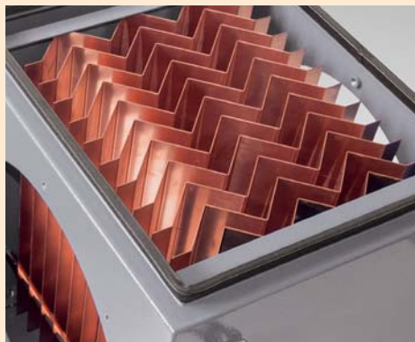
Vista detallada de las laminas de cobre (aprox. 17 kg contenido en cobre)
