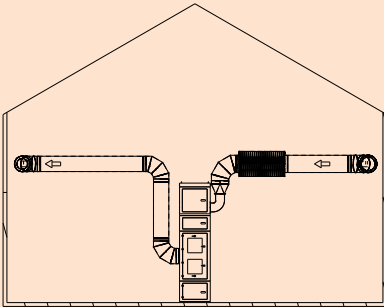
Ejemplo de utilización: Sistema PushPull en la nave
